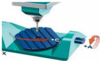
图 1 摇篮式五轴机床
