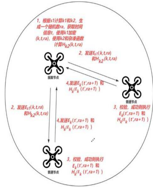
图2 无人机集群簇首节点与普通节点双向认证及密钥同步流程
