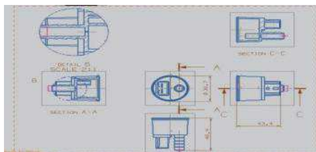
图 3 塑件的二维图
