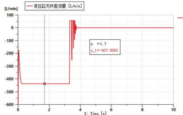
图 4 液压缸无杆腔流量
