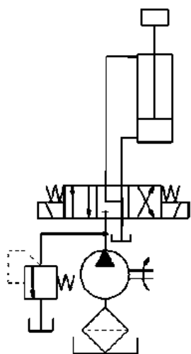
图 1 液压回路 1
