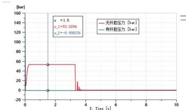
图 3 有杆腔和无杆腔压力
