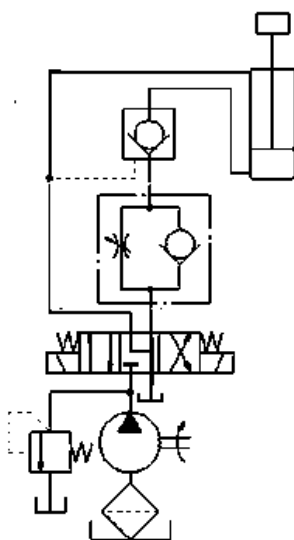
图5 采用液控单向阀的平衡回路
