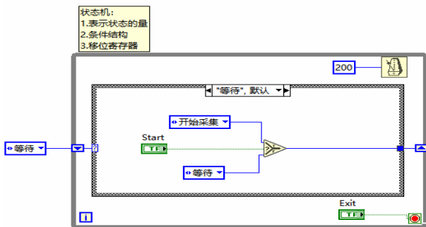
图 2 温度采集系统程序图
