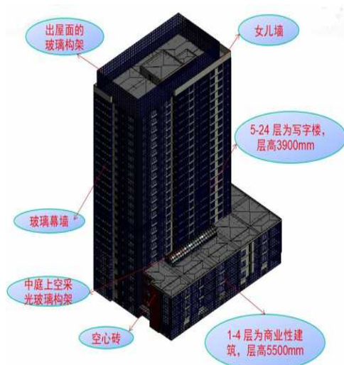
图 3.1 旺景国际广场 BIM
