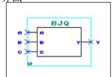
图 4 三人表决器电路符号
