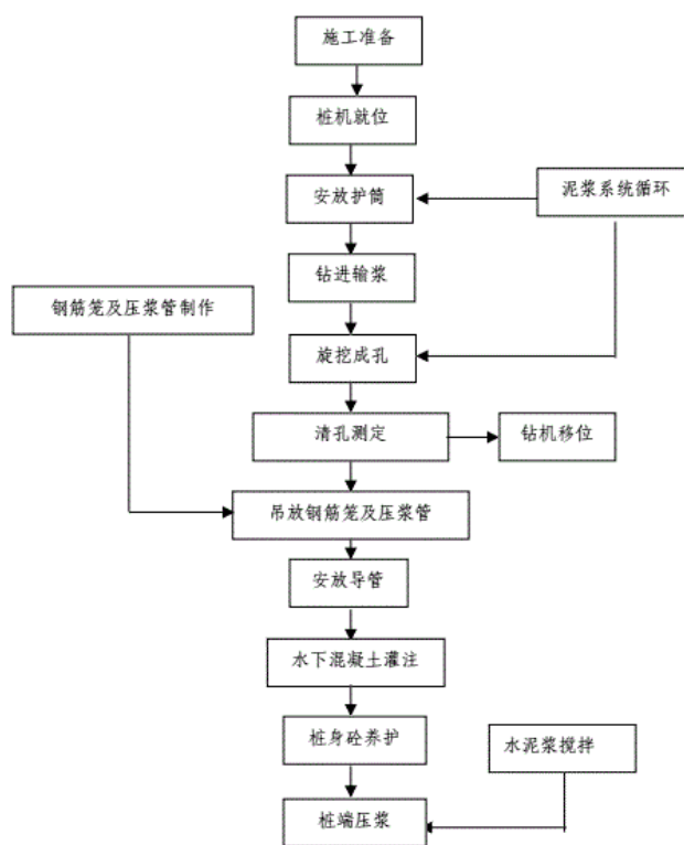
图 1 钻孔灌注桩施工工艺流程图
