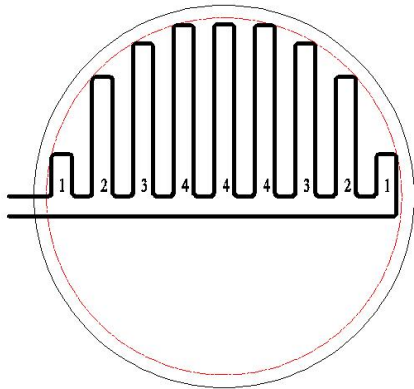
图 3 毡房底部辐射供热管道示意图
