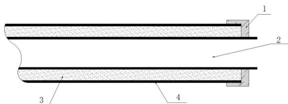
1-封头 2-水管 3-相变微胶囊 4-套管
