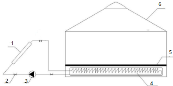
1-太阳能集热器 2-控制阀门 3-水泵 4-盘管 5-面层 6-毡房主体 图 2 太阳能—热水供暖系统示意图
