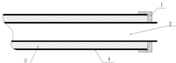
1-封头 2-水管 3-相变微胶囊 4-套管
