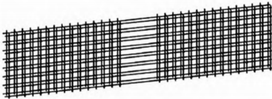
图 1 后浇带钢筋绑扎基本形式
