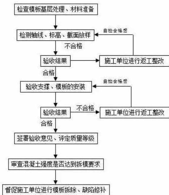
图1 土建监理流程
