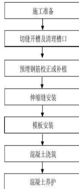
图 1 公路桥梁伸缩缝安装施工方法
