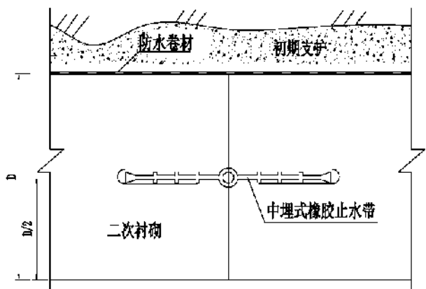
图 3 为施工缝止水带设计图纸
