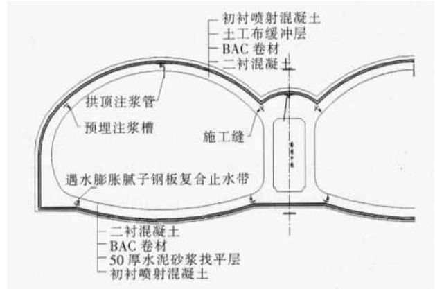
图 2 为公路桥梁隧道建设防水施工
